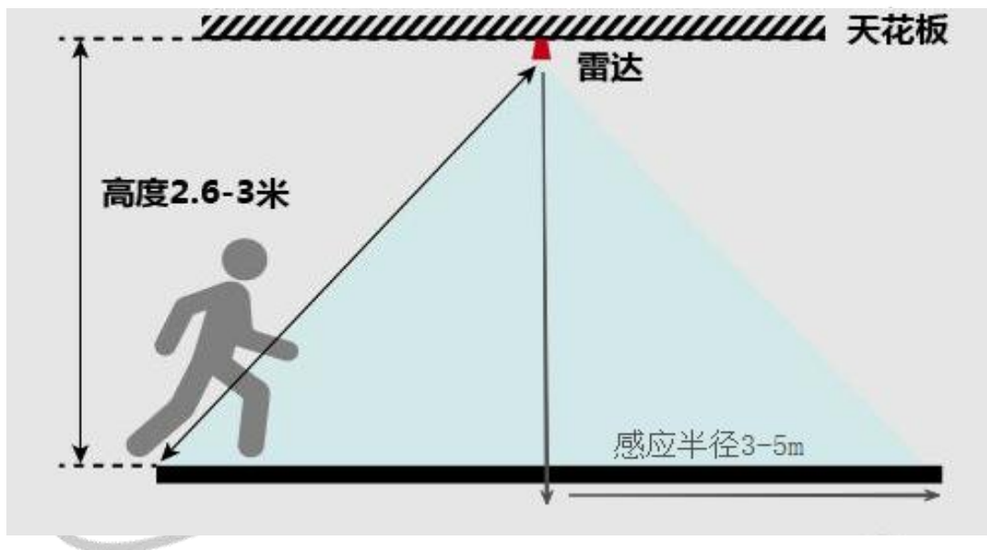
挂高探测图（距离设置 6m）
