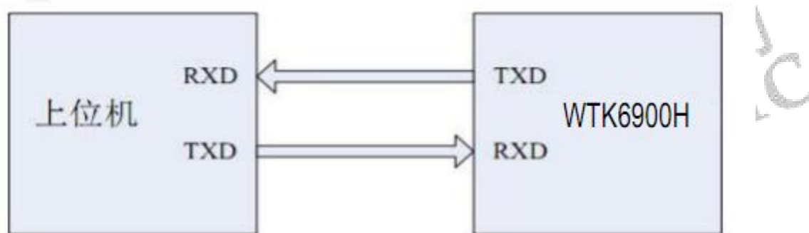
图表 3- WTK6900H 芯片 UART 接口连接示意图
