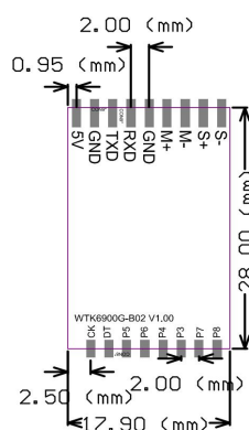
图表 2 - WTK6900G-B02 模块尺寸图
