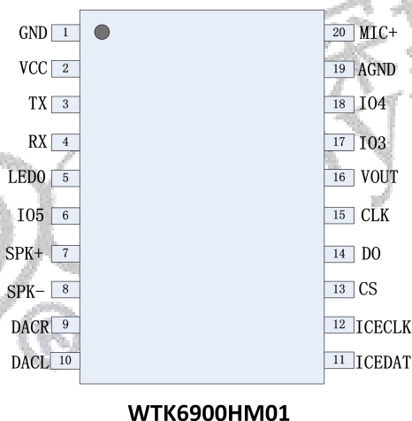
图表 2 - WTK6900HM01 模块管脚分布
